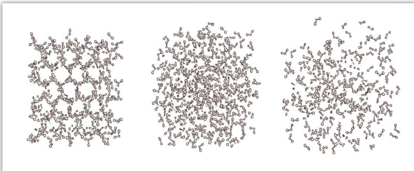
Obr. 1 Zleva struktura ledu, vody a páry
